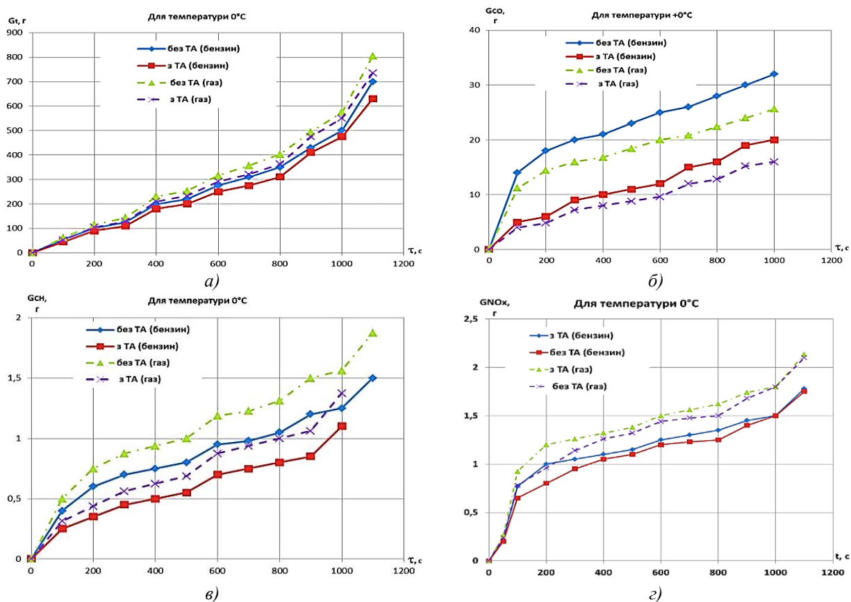
Рис. 5. Розрахункові залежності при здійсненні прогріву двигуна ТЗ в русі в режимах їздового циклу: сумарна витрата палива, г (а); сумарні викиди CO , г (б); сумарні викиди SpHt , г (в); сумарні викиди NOx , г (г)
