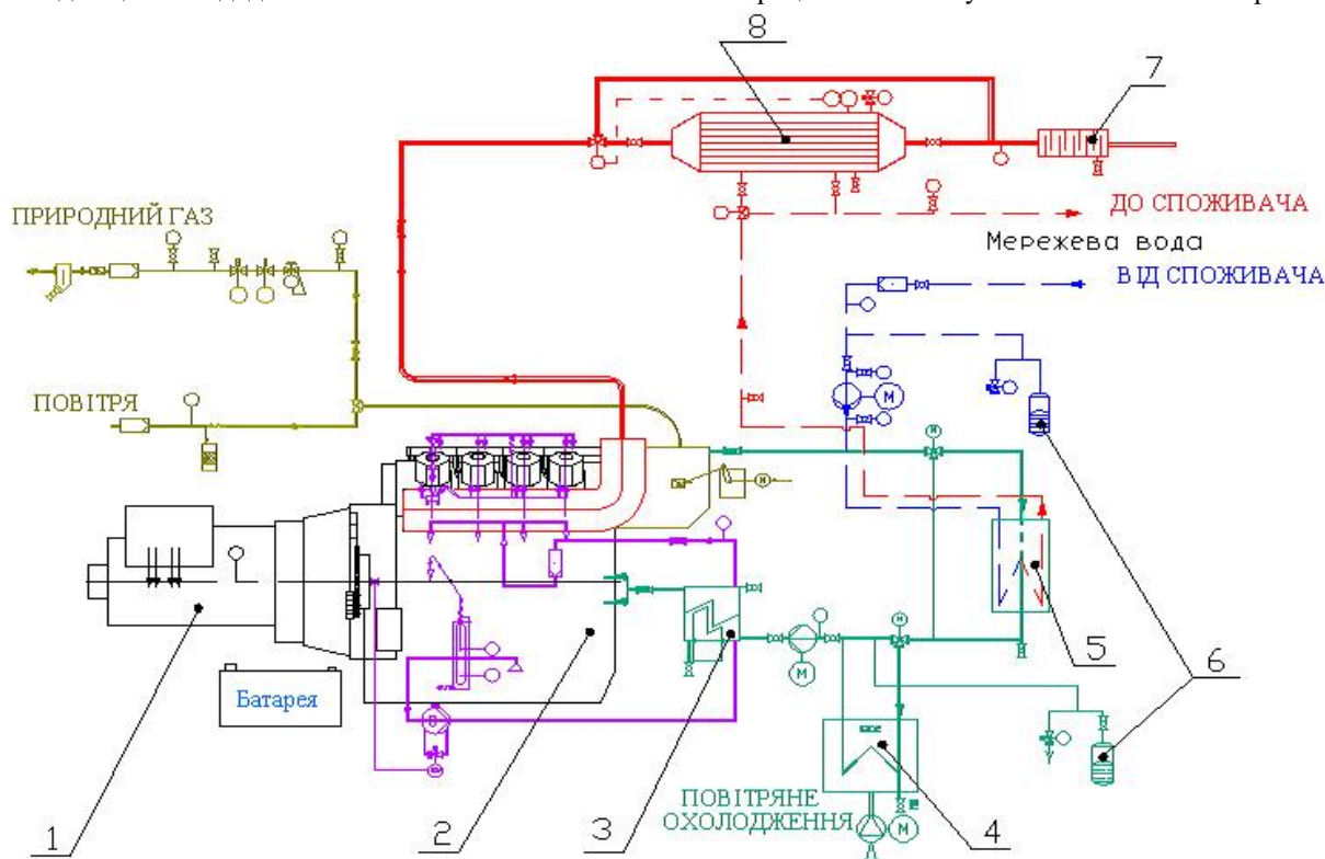
Рис. 1. Принципова схема когенераційної газової установки :
