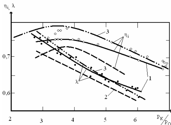
Рис. 7. Зависимость коэффициента подачи \lambda и индикаторного КПД \eta_i ТНУ от отношения давлений P_K / P_O : 1 – смесь; 2 – хладагент R12; 3 – хладагент R142B
