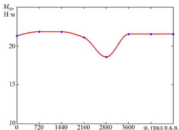
Рис. 7. Зміна середнього крутного моменту при плавному відключенні трьох циліндрів
