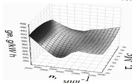
Рис.2. Зависимость g_e = f_2(x)
