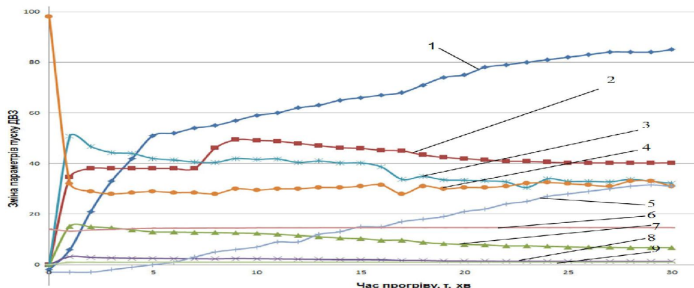
Рис. 6. Зміна основних діагностичних параметрів ДВС, що характеризують процеси його пуску і прогріву: 1 – температура охолоджуючої рідини, t , ^{\circ}\text{C} ; 2 – температура каталізатора ( \times 10 ), t , \text{K} ; 3 – абсолютне значення навантаження; 4 – тиск у впускному колекторі; 5 – температура повітря на впуску, t , ^{\circ}\text{C} ; 6 – співвідношення компонентів паливо-повітряної суміші :1; 7 – частота обертання ( \times 100 ), \text{хв}^{-1} ; 8 – витрата палива ( \text{л}/\text{год} ); 9 – коефіцієнт надлишку повітря
