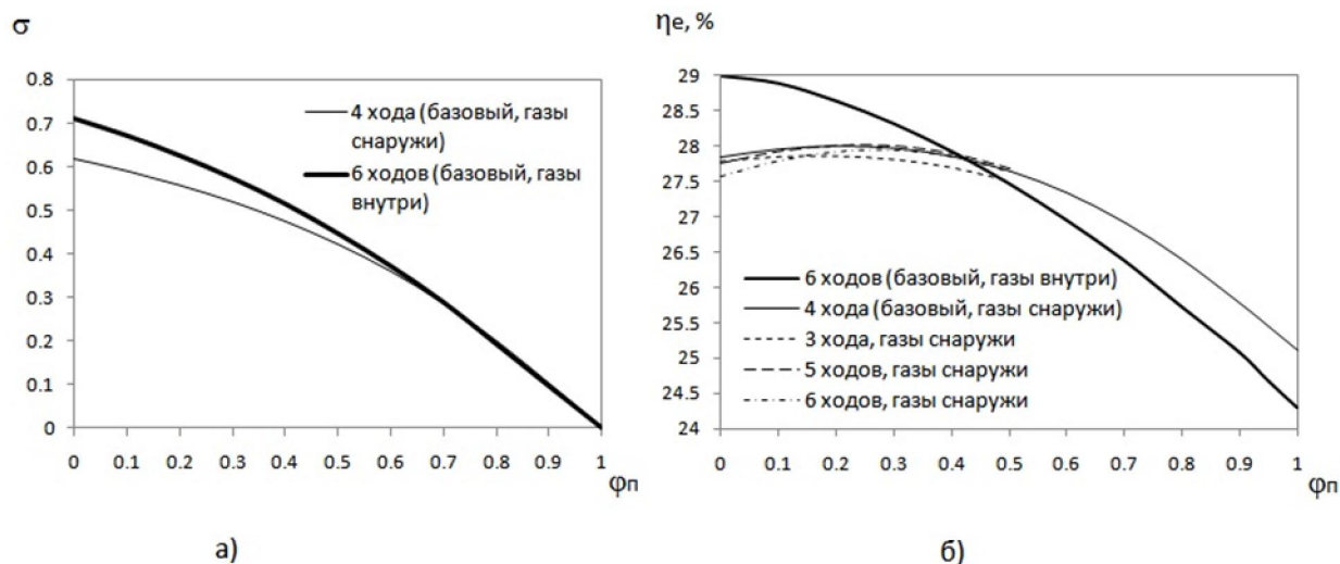
Рис. 3. Показатели эффективности регенератора и установки в зависимости от доли перепуска горячих газов мимо регенератора: а – степень регенерации; б – эффективный КПД ГТУ
