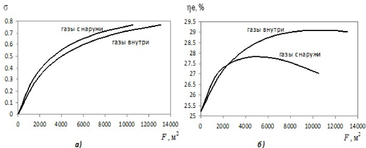
Рис. 2. Показатели эффективности регенератора и установки в зависимости от площади поверхности регенератора а – степень регенерации; б – эффективный КПД ГТУ
