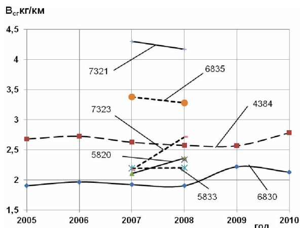
Рис.3. Среднегодовой удельный расход топлива тепловозами ЧМЭ-3 в кг на км пробега
