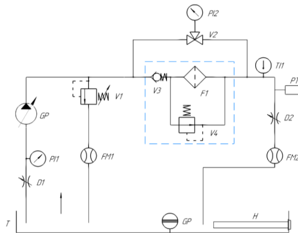
Рис. 4. Гідравлічна схема стенду
