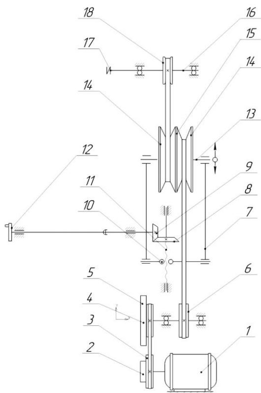
Рис. 2. Кінематична схема приводу стенду: 1 – електродвигун; 2, 3, 4, 5, 6 – шків; 7 – рамка; 8, 9 – шестерні; 10 – гайка; 11, 13, 16 – вали; 12 – маховичок; 14, 15 – шків варіатору; 17 – сполучна муфта
