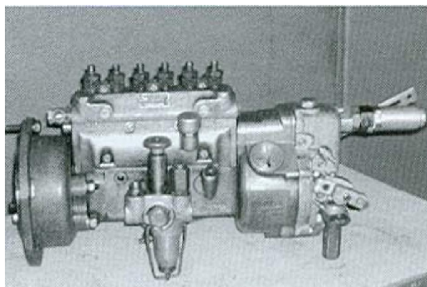
ПНВТ WSK для газодизеля
