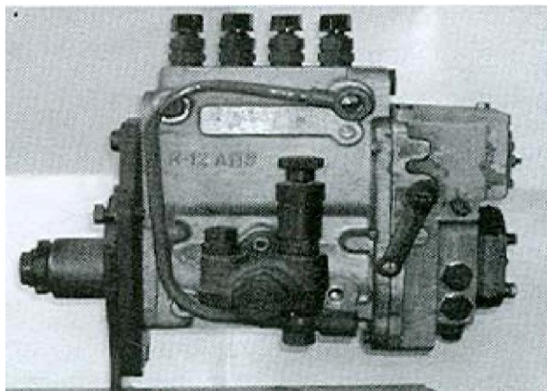
ПНВТ УТН-6Г з гідравлічним регулятором
