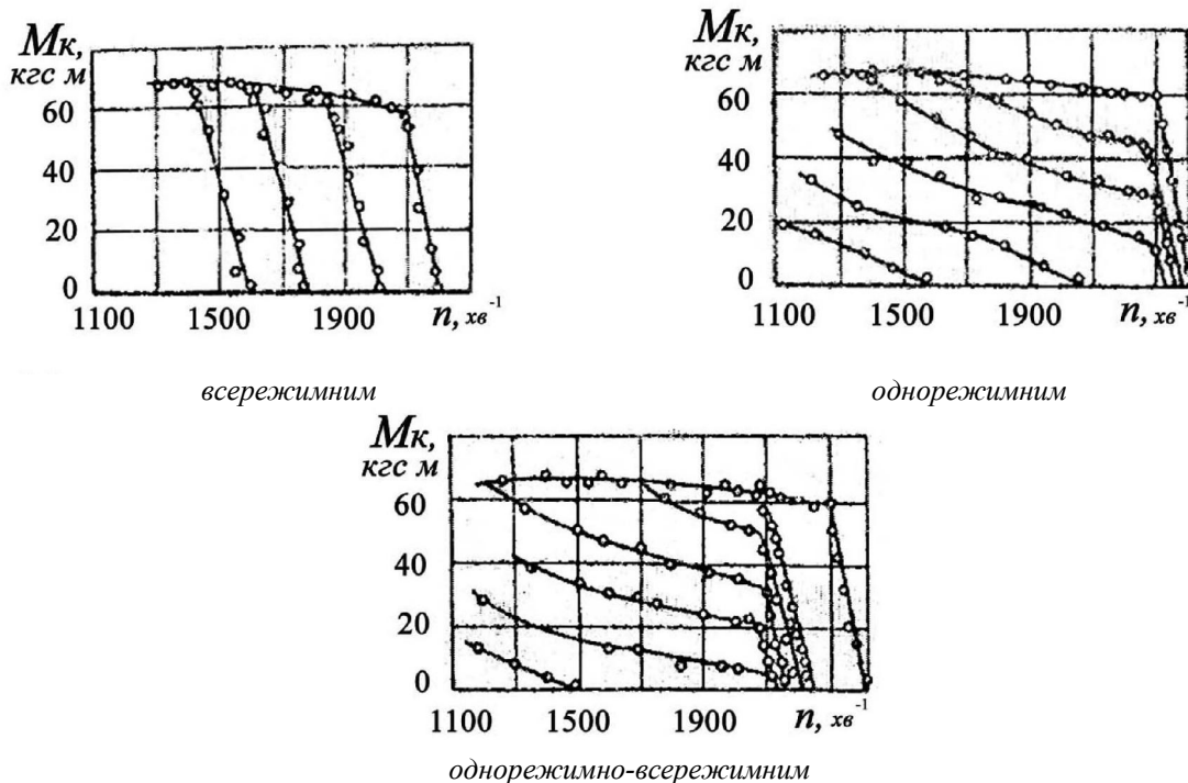
Рис. 3. Приклади швидкісних характеристик дизеля ЯМЗ-236 з гідравлічними регуляторами
