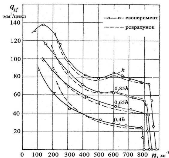
Рис. 1. Швидкісні характеристики паливоподачі роторного паливного насосу РТНГ-2М
