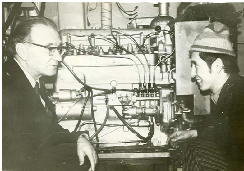
Кінт Євгенович з аспірантом Сатибалдієвим Г. в процесі випробування паливного насоса високого тиску з гідравлічним регулятором
