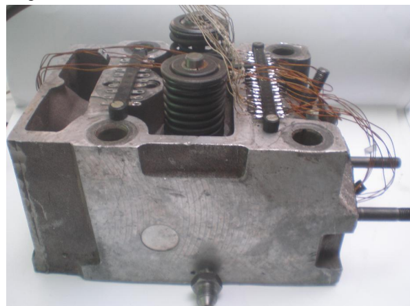
Рис.2. Опытная ГЦ дизеля КамАЗ
