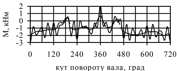
Рис. 5. Згинальні моменти в перерізі 4-ї щоки;
