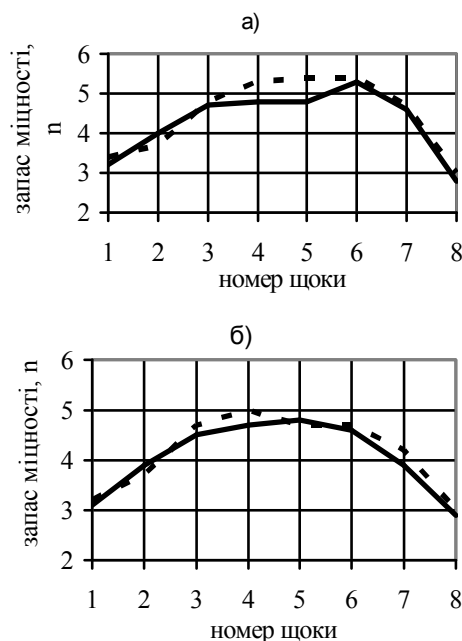
Рис. 3. Запаси міцності для розрахунків 2-го етапу; розрахунки: а – ——— 1, - - - - 6, б – ——— 5, - - - - 7
