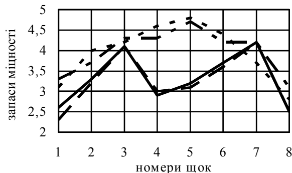
Рис. 4. Запаси міцності для розрахунків 3-го етапу;
