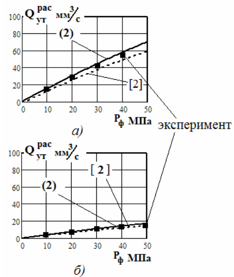
Рис. 3 Расчетные и экспериментальные зависимости Q_{ут}^{рас} = f(\delta_n, P_\phi) полученные для: а) – распылителя №1; б) – распылителя №2 (см. табл. 1)
