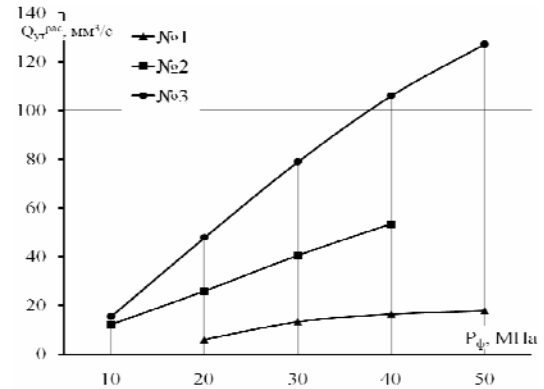
Рис. 2 Экспериментальные зависимости
