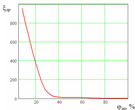
Рис. 3. Залежність місцевого опору \xi_{др} від кута відкриття дросельної заслінки \phi_{др}
