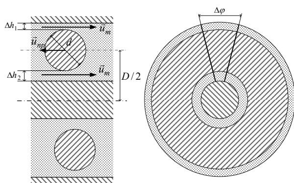
Рис. 2. Схема течения жидкости при движении пружины в тесном канале
